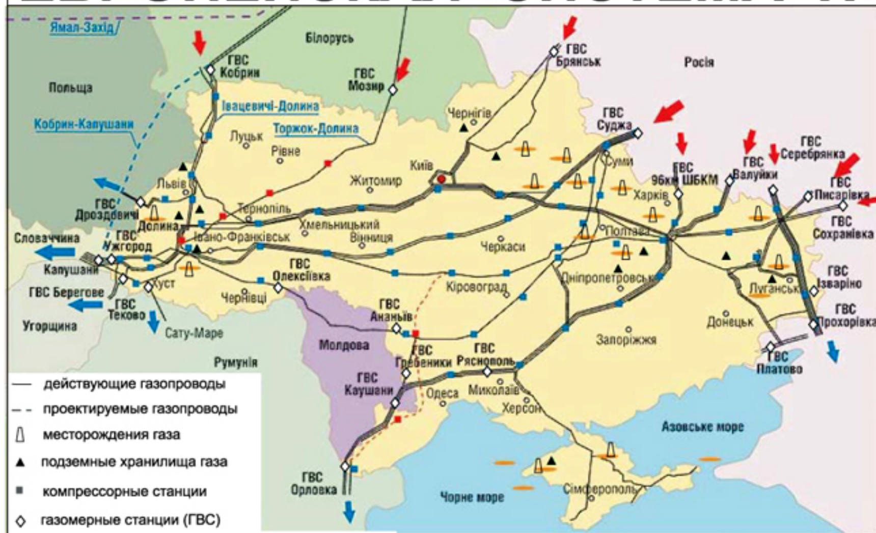
Сеть транзитных газопроводов Украины Источник: http://kontrakty.com.ua
